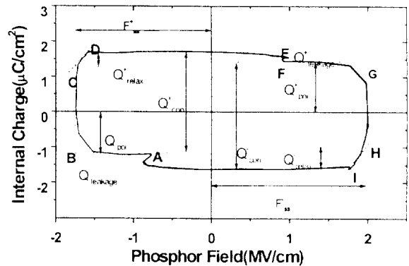
그림 9. TFEL 소자에 인가되는 쌍극성 파형(a). (b) 실제 ZnS:Pr, Ce 소자에 대한 Qint-Fp loop. 각각의 표시점은 (a) 그림의 표시점에 해당함[16].
