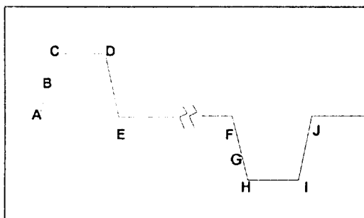
그림 9. TFEL 소자에 인가되는 쌍극성 파형(a). (b) 실제 ZnS:Pr, Ce 소자에 대한 Qint-Fp loop. 각각의 표시점은 (a) 그림의 표시점에 해당함[16].
