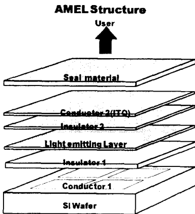
그림 13. Active matrix TFEL(AMEL) 소자의 구조.
