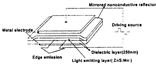
그림 11. 측면 방출광을 이용한 Edge emitter
