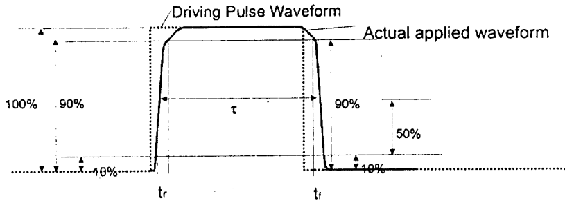
그림 7. 이상적인 구동파형과 실제 소자에 인가되면서 변형된 실제파형.
