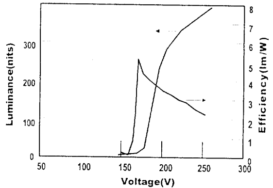
그림 4. ZnS:Mn TFEL 소자의 휘도-인가전압 및 발광효율-인가전압 특성곡선.
