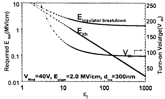
그림 12. 상하 절연층의 유전상수값과 소자의 발광 개시전압과의 관계.
