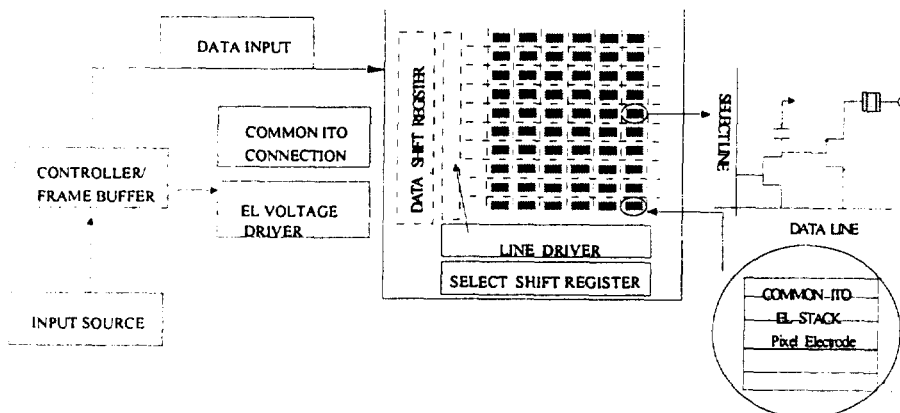
그림 14. AMEL 디스플레이에 대한 block diagram.
