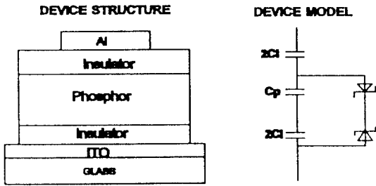
그림 5. TFEL 소자와 소자에 대한 등가회로 모델.
