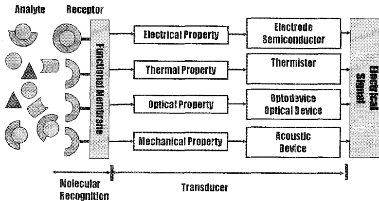
<그림 2-1> 신호변환기(Transducer)의 개념도
