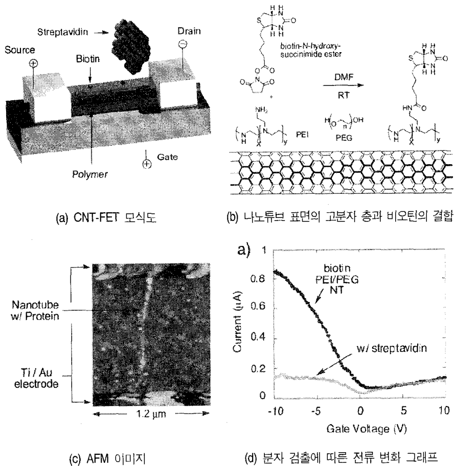
<그림 3-10> 스트렙토아비딘과 비오틴의 반응을 이용한 CNT-FET
