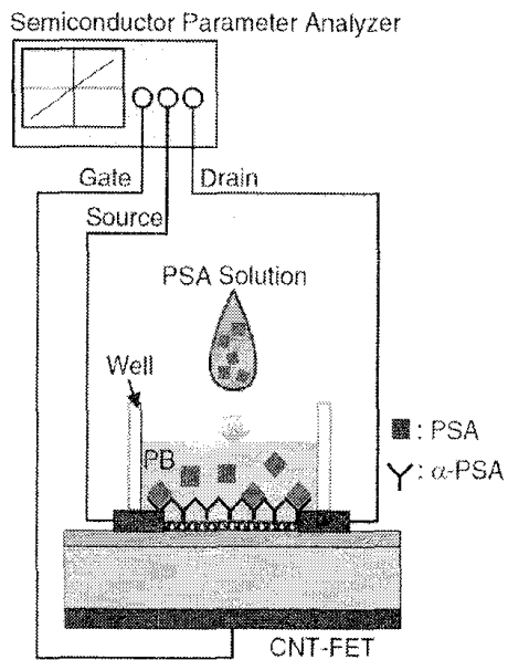
<그림 3-13> 항원-항체 반응 장비
