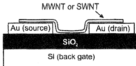
<그림 2-4> CNT-FET 모식도
