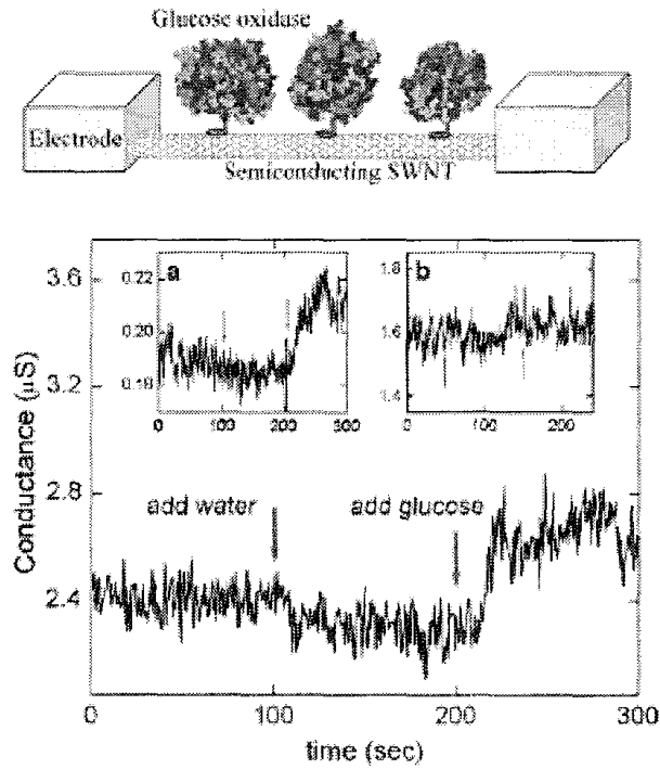
<그림 3-11> 글루코즈옥시이드를 이용하여 탄소나노튜브를 처리 한 pH 센서용 CNT-FET
