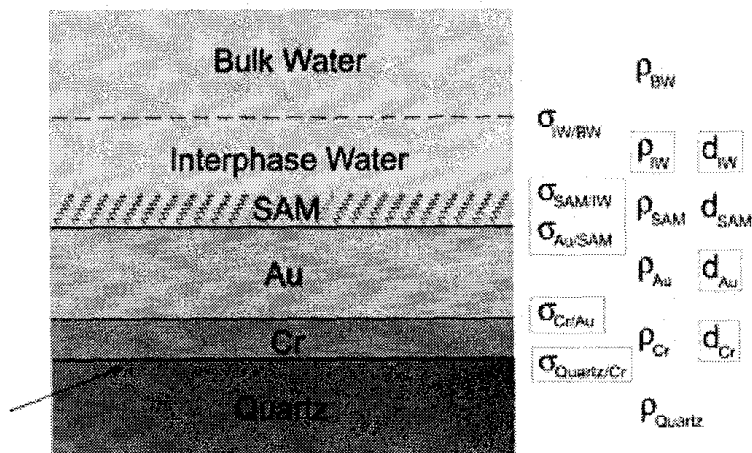
&lt;그림 3-3&gt; 독일의 Steitz 그룹의 연구에서 사용된 다층막 구조에 대한 개략도
