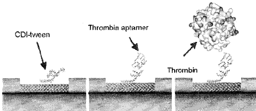
<그림 3-17> CNT-FET를 이용한 앵타머 센서
