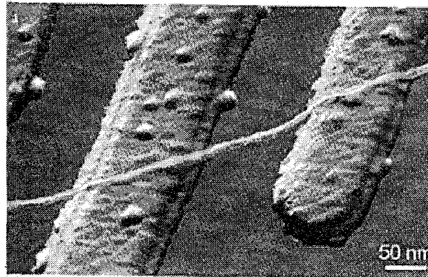
<그림 2-5> CNT-FET AFM 이미지(Nature 발췌)
