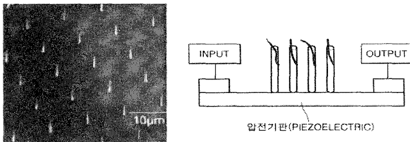
<그림 3-16> 수직방향배열 탄소나노튜브 바이오 칩
